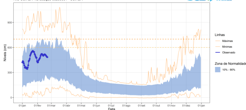
Níveis observados e comparação com histórico RIO SÃO LOURENÇO na estação 66460000 - ACIMA DO CÓRREGO GRANDE
