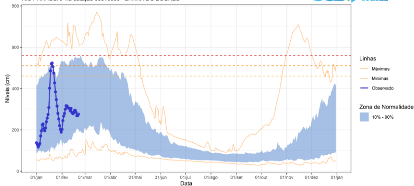
Níveis observados e comparação com histórico RIO PARAGUAI na estação 66070004 - CÁCERES (DNPVN)
